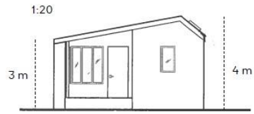
Facadeopstalt; sadeldagsvariant, tosidet hældning
